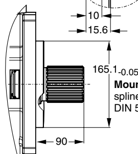
Output: splined shaft W 50x2x24x9g DIN 5480
