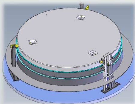
Locklyft Ø 15,5m, 130 ton
